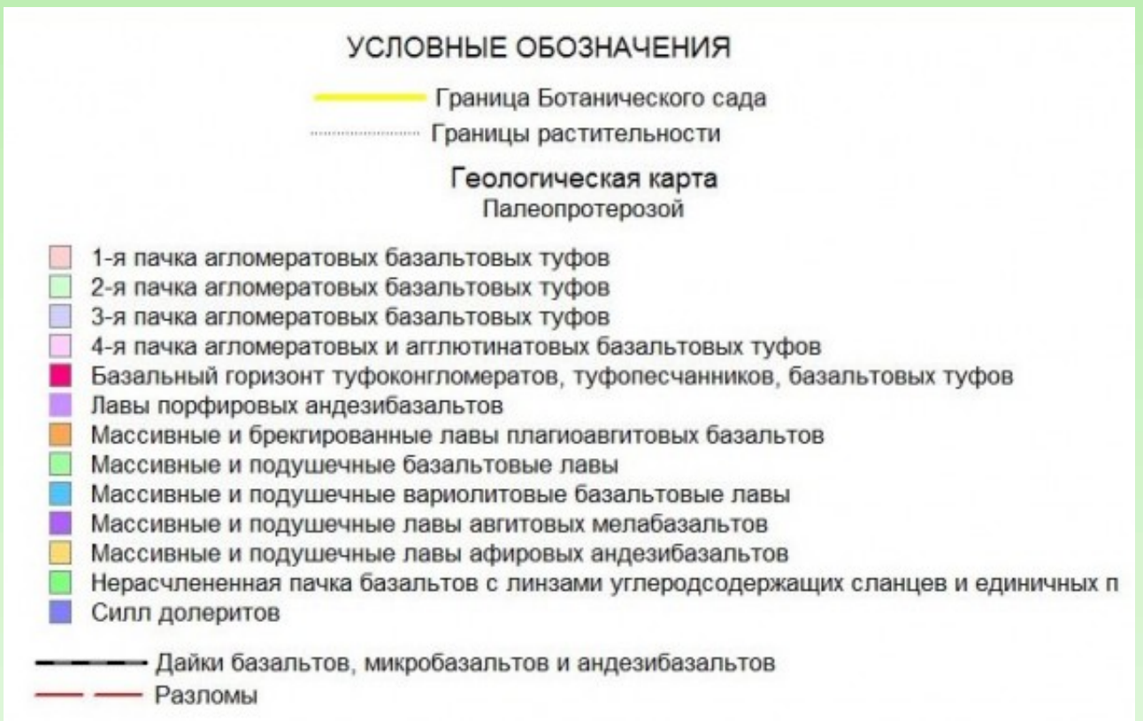
Рис. 5. Геологическая карта территории БС ПетрГУ. Палеопротерозой.
