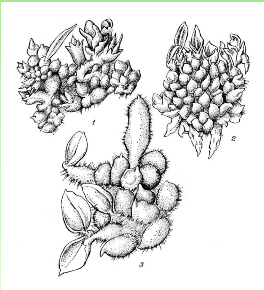
Протокормы орхидных.
