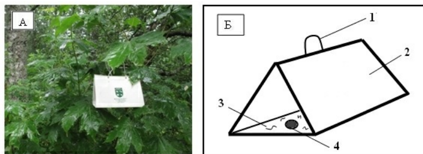
Рис. 3. А. – Установка дельтовидной ловушки на территории Ботанического сада ПетрГУ. Б. – Схема дельтовидной ловушки. Обозначения: 1 – подвес для крепления ловушки, 2 – картонный корпус, 3 – клейкая основа, 4 – диспансер с феромоном.
