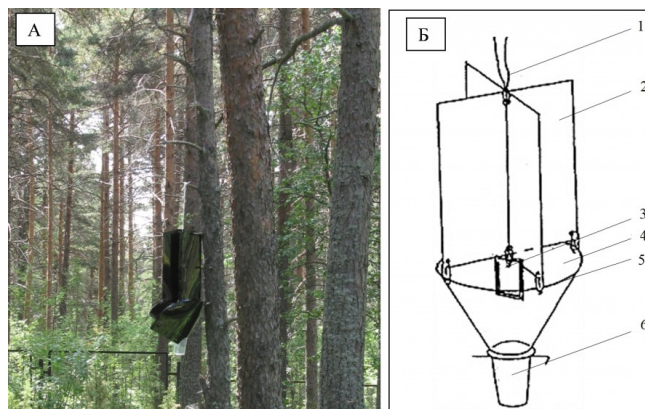
Рис. 2. А. – Расположение барьерно-вороночной ловушки на территории Ботанического сада ПетрГУ. Б. – Схема устройства барьерно-вороночной ловушки. Обозначения: 1 – подвес для крепления ловушки, 2 – крестообразный экран, 3 – диспансер с феромоном, 4 – воронка, 5 – стакан (накопитель насекомых).
