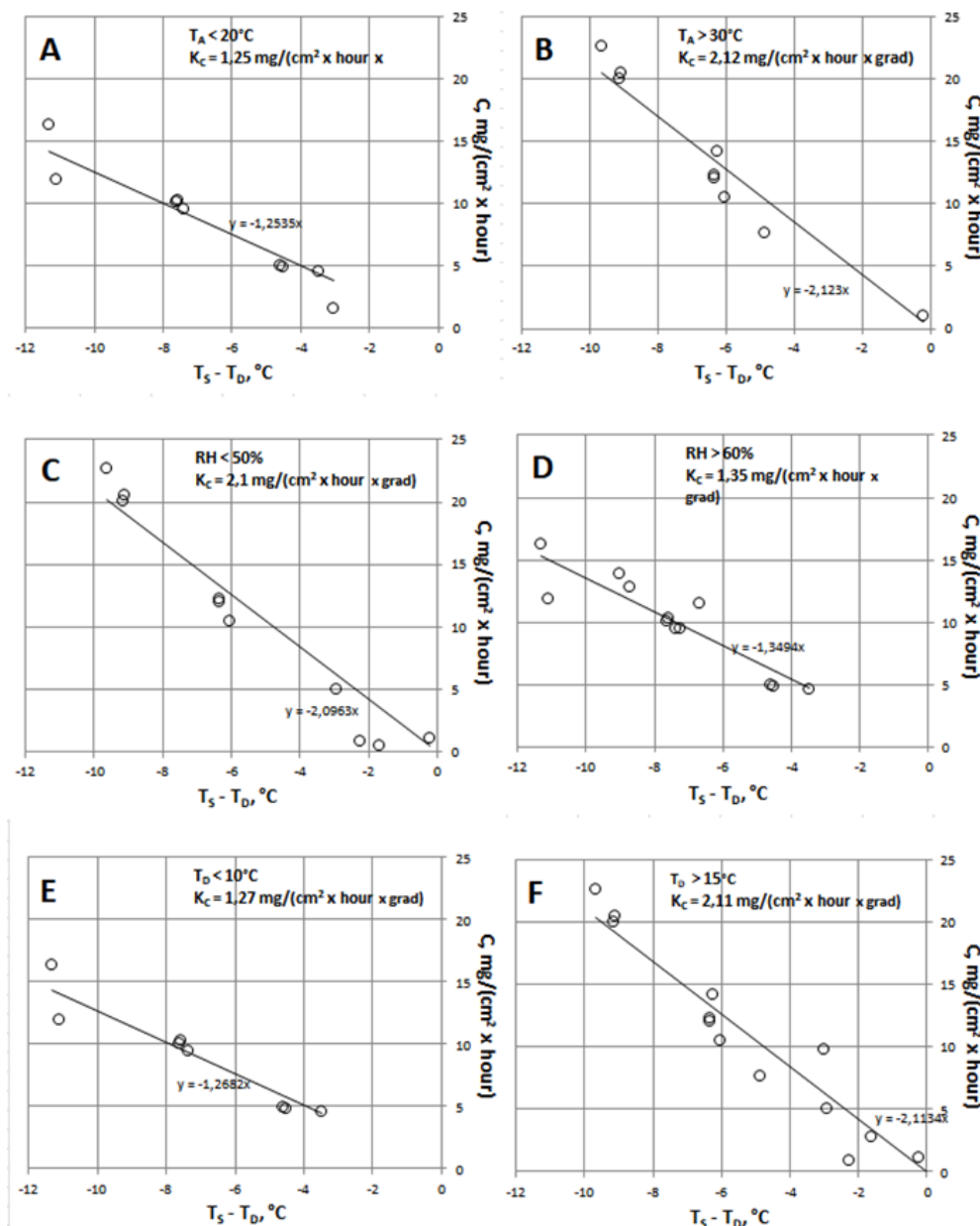
Рис. 3. Зависимость эффективности конденсации воды ( C ) от снижения T_S относительно T_D при T_A < 20^\circ\text{C} (A) и T_A > 30^\circ\text{C} (B), при RH < 50\% (C) и RH > 60\% (D), при T_D < 10^\circ\text{C} (E) и T_D > 15^\circ\text{C} (F).
